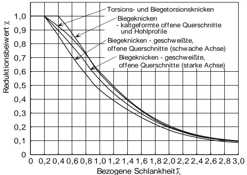
Abbildung 5.1 Knickspannungslinien für Biegeknicken, Drill- und Biegedrillknicken
