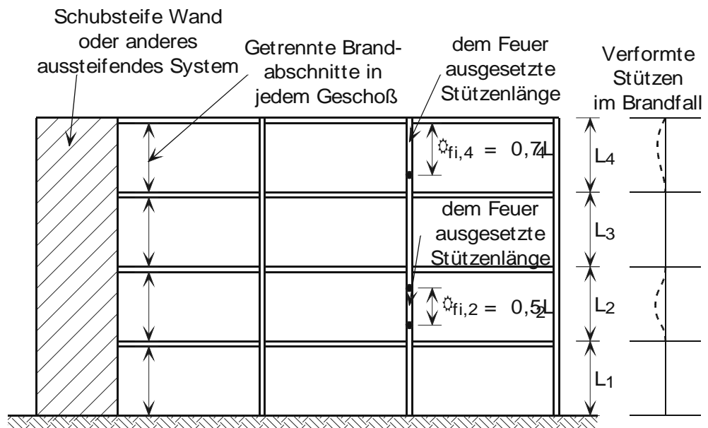
Abbildung 7.1 Knicklängen l_{fi} von Stützen in ausgesteiften Rahmen
