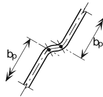
c) Nennweite b_p für einen Steg ( b_p \equiv geneigte Höhe s_w )
