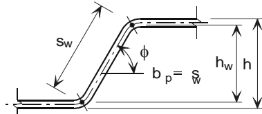
c) Nennweite b_p für einen Steg ( b_p \equiv geneigte Höhe s_w )
